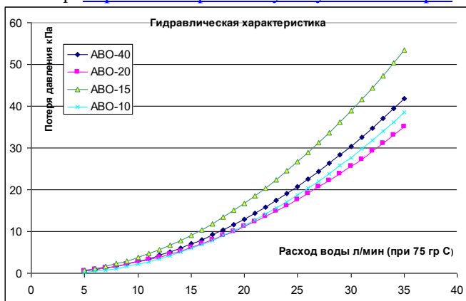
Рис. 1 - Гидравлические характеристики
